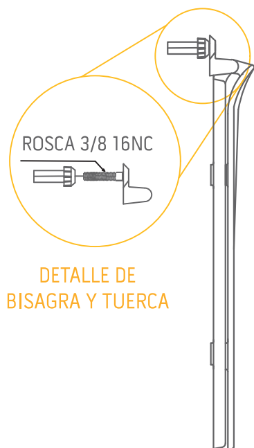
VISTA LATERAL
