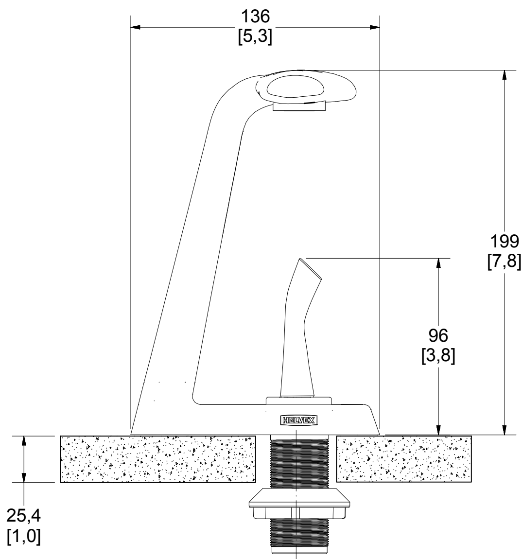
Medidas Referenciales / Estimated Dimensions, Acot. mm [pulg.] / Dim. mm [inch.]
