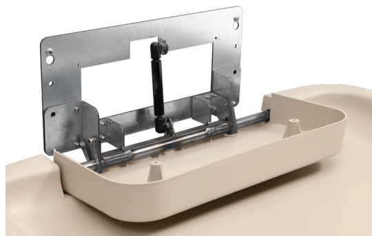
Marco de acero para mayor resistencia e instalación sencilla.
