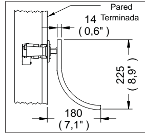
Acot.mm.(pulg) / Dim.mm.(in)
