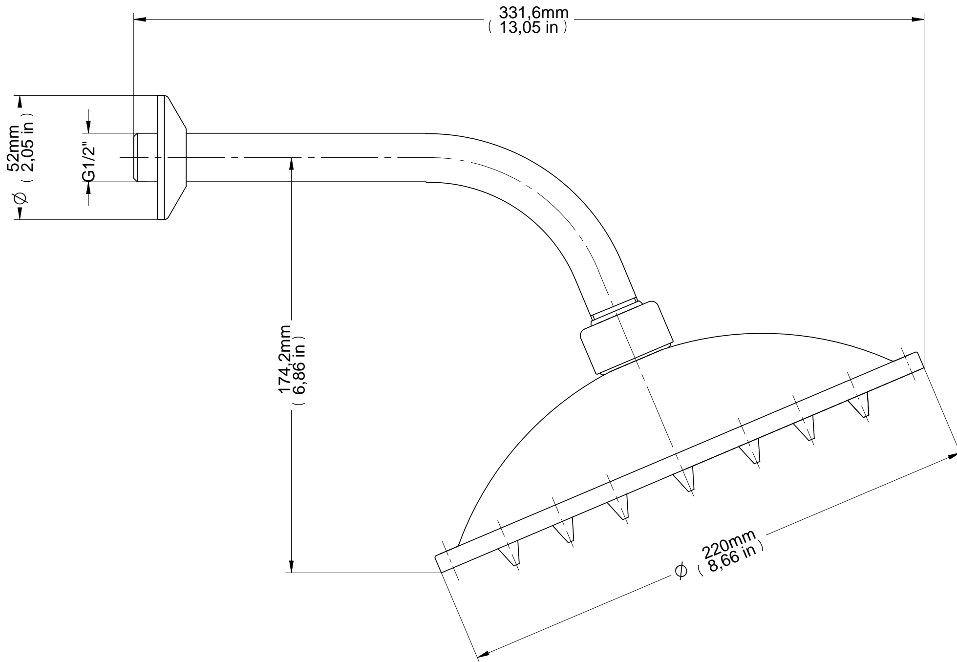
CHUVEIRO LINHA BILBAO SHOWER - 1/2" - BILBAO DUCHA - 1/2" - BILBAO
